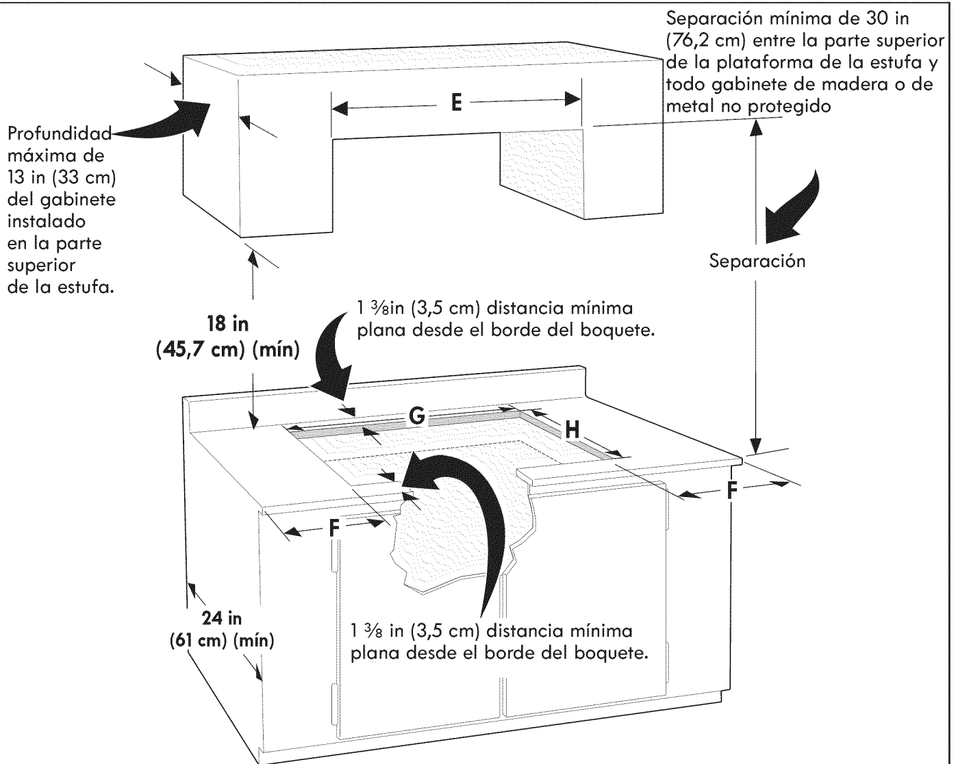
Figura 2 – DISEÑO DEL GABINETE
