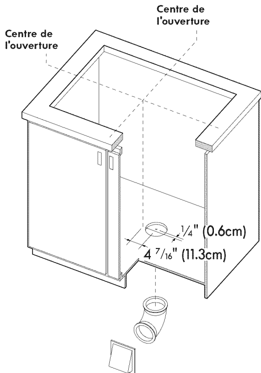
Figure 11 – MODÈLE 36" SORTIE D'ÉCHAPPEMENT VERS LE BASE
