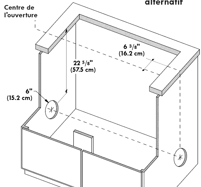
Figure 13A – MODÈLE 30" SORTIE DE CONDUITS ALTERNATIFS
