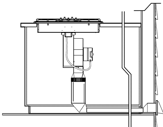
Figure 6 – CONDUIT SUR LE PLANCHER
