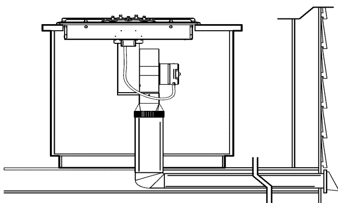
Figure 7 – CONDUIT À TRAVERS LE PLANCHER 34
