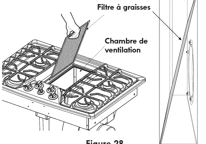
Figure 28 EMPLACEMENT DU FILTRE À GRAISSES – MODÈLE 30"
