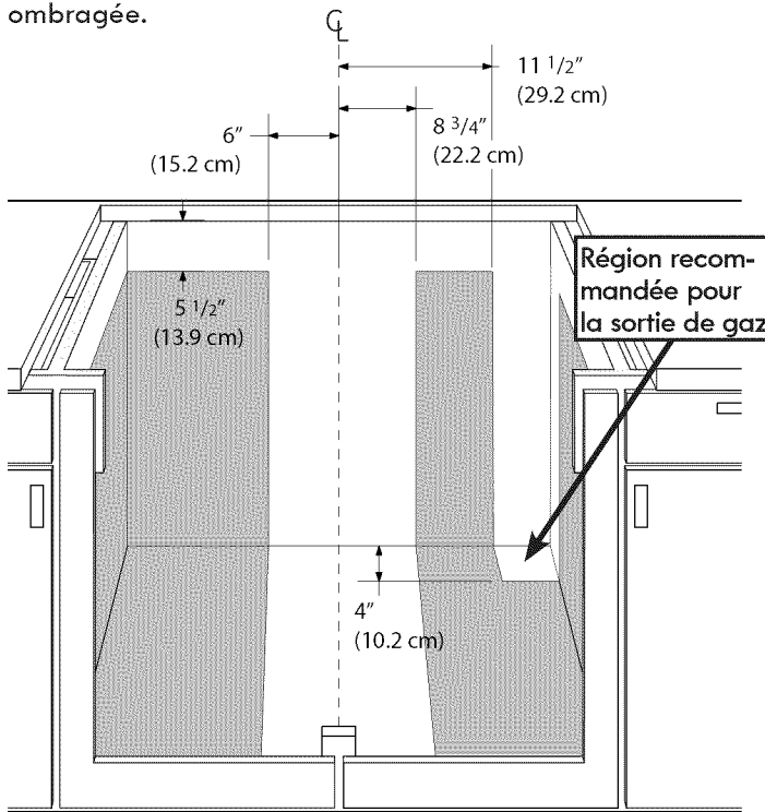
Figure 3A - MODÈLE 36'' DIMENSIONS D'INSTALLATION DE LA PRISE DE COURANT
