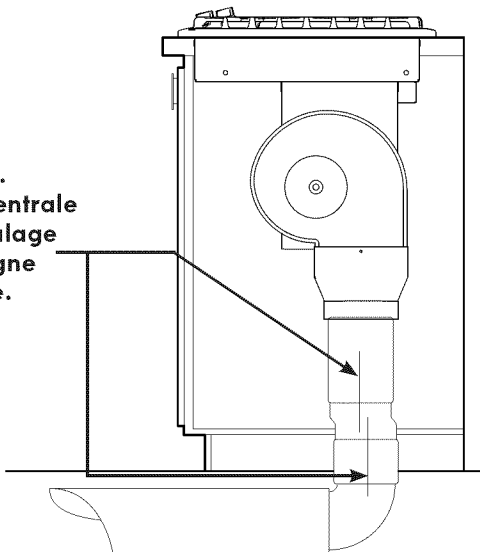
Figure 14 – ALIGNEMENT DU CONDUIT
