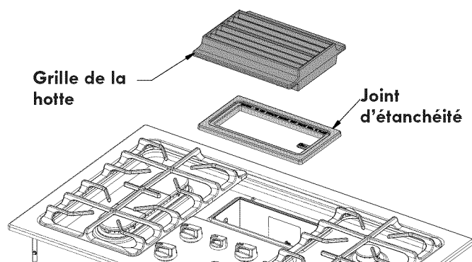
Figure 33 – MODÈLE 36" EMPLACEMENT DE LA GRILLE DE HOTTE ET DU JOINT D'ÉTANCHÉITÉ
