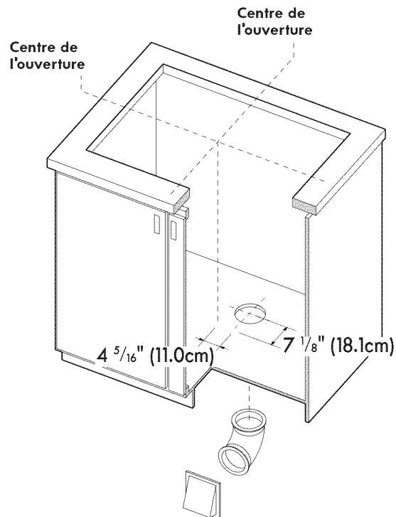
Figure 9 – MODÈLE 30" SORTIE D'ÉCHAPPEMENT VERS LE BAS
