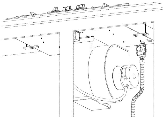
Figure 25 – ATTACHEMENT PHYSIQUE DE LA CANALISATION DE GAZ À LA SURFACE DE CUISSON
