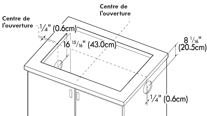
Figure 12 – MODÈLE 36" SORTIE D'ÉCHAPPEMENT LATÉRAL
