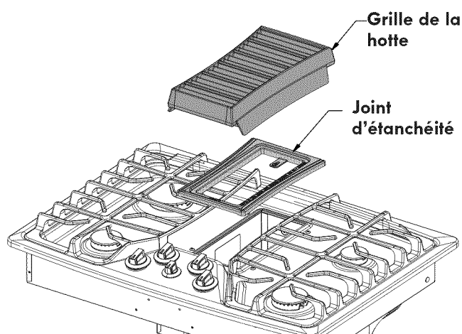
Figure 32 – MODÈLE 30" EMPLACEMENT DE LA GRILLE DE HOTTE ET DU JOINT D'ÉTANCHÉITÉ
