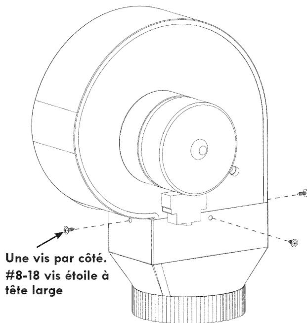
Figure 20 – ATTACHEZ LA TRANSITION À LA SOUFFLERIE
