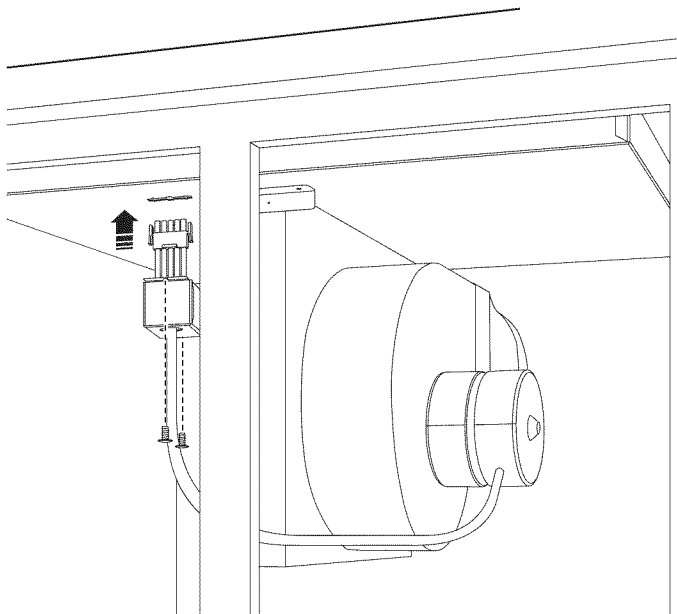
Figure 23 – CONNECTEZ LA SOUFFLERIE À LA TABLE DE CUISSON
