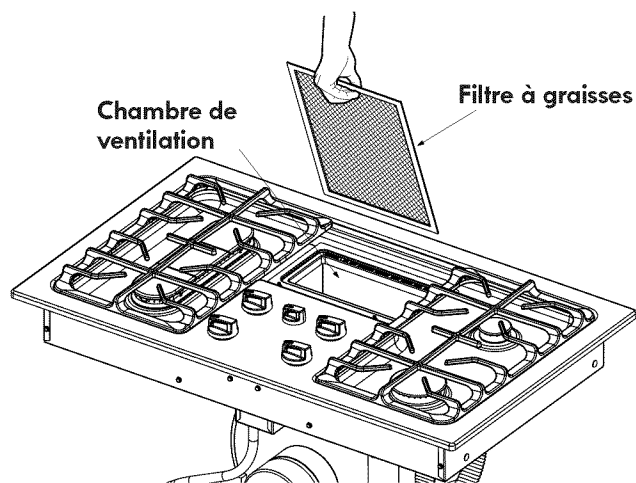
Figure 29 EMPLACEMENT DU FILTRE À GRAISSES – MODÈLE 36"
