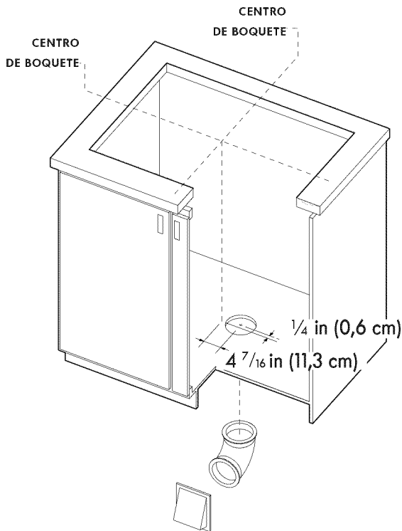
Figura 11 – MODELO DE 36 PULGADAS ORIFICIO DE LA DUCTERÍA EN EL FONDO
