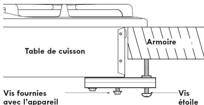
Figure 17 – FIXEZ L'APPAREIL AU COMPTOIR
