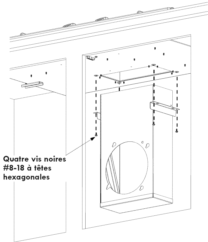
Figure 19 – MODÈLE 36" – INSTALLATION DU PLÉNUM À LA PLAQUE DE CUISSON
