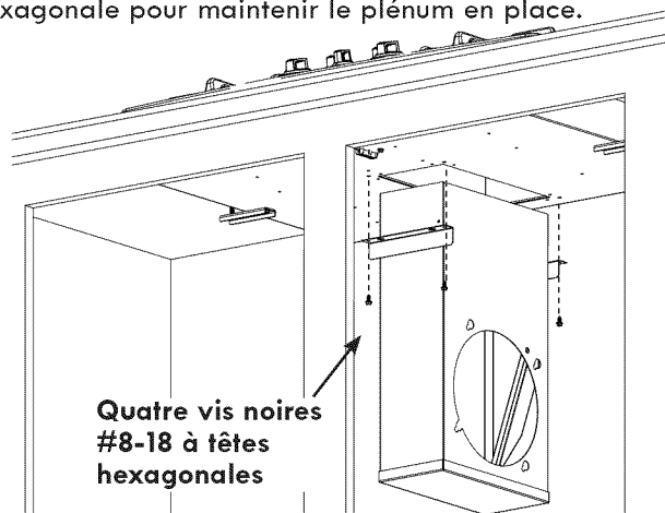
Figure 18 – MODÈLE 30" – INSTALLATION DU PLÉNUM À LA PLAQUE DE CUISSON
