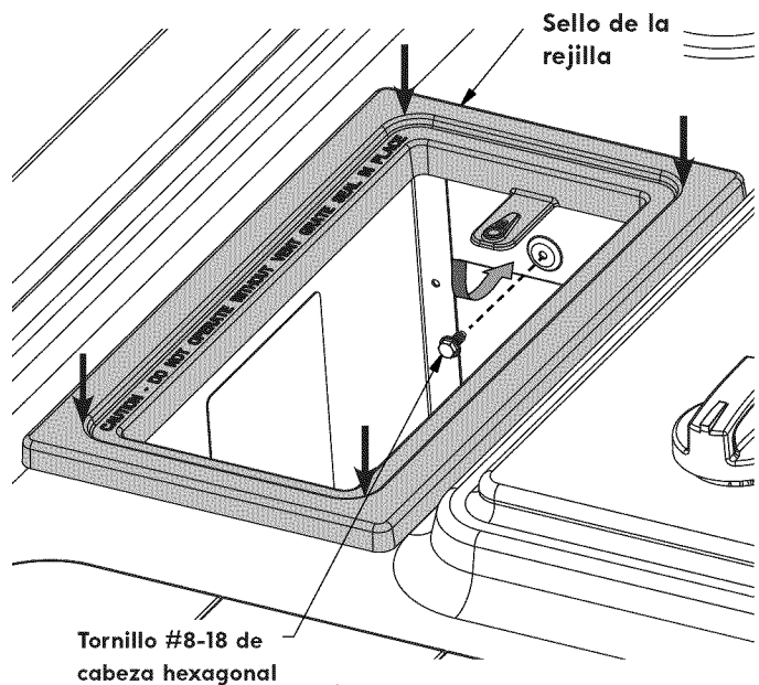
Figura 31 FIJACIÓN DEL SELLO DE LA REJILLA DE VENTILACIÓN – MODELO DE 36 PULGADAS
