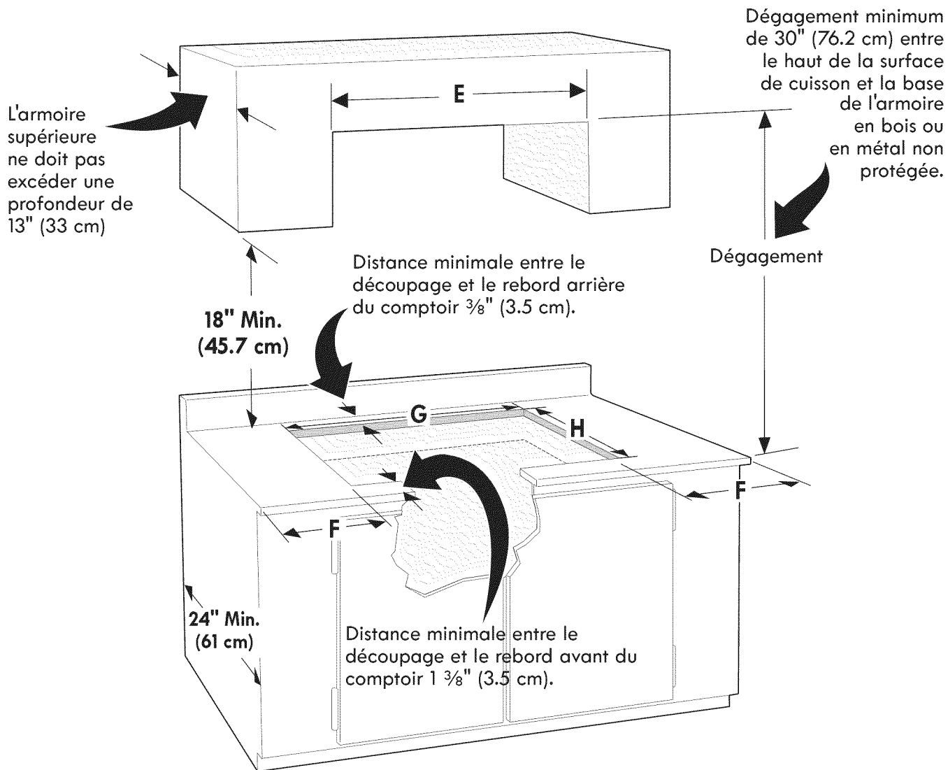
Figure 2 – DÉCOUPAGE DU DESSUS DU COMPTOIR
