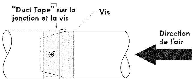
Figure 5 – «DUCT TAPE» SUR LA JONCTION ET LA VIS
