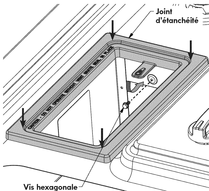
Figure 31 – MODÈLE 36" EMPLACEMENT DU JOINT D'ÉTANCHÉITÉ
