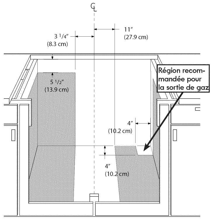
Figure 3B - MODÈLE 30'' DIMENSIONS D'INSTALLATION DE LA PRISE DE COURANT
