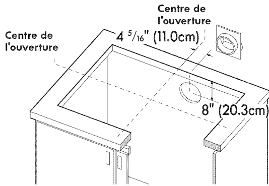
Figure 10 – MODÈLE 30" SORTIE D'ÉCHAPPEMENT VERS L'ARRIÈRE
