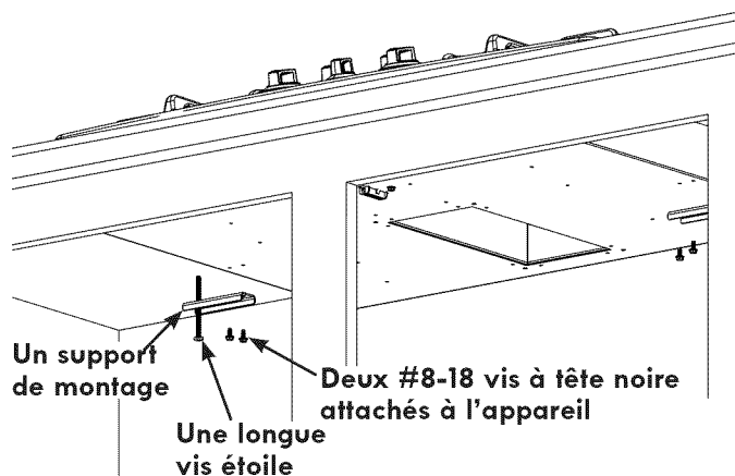
Figure 16 – FIXEZ LES DEUX SUPPORTS DE MONTAGE
