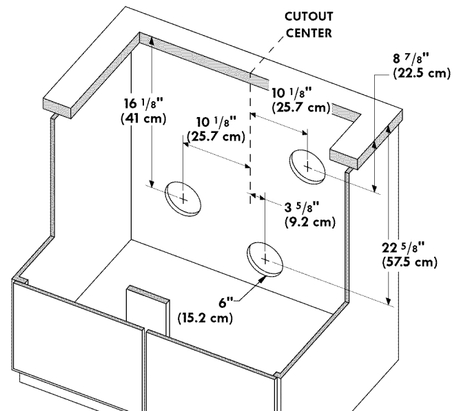
Figure 13B – MODÈLE 36" SORTIE DE CONDUITS ALTERNATIFS
