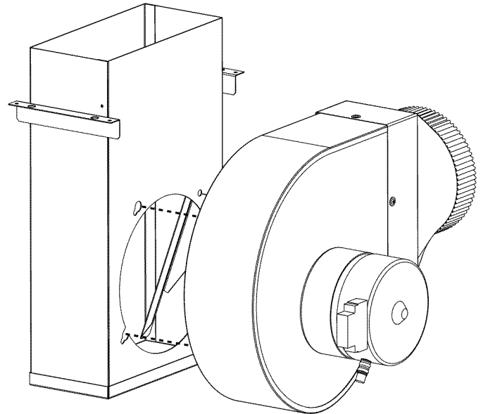
Figure 21 – ATTACHEZ LA SOUFFLERIE AU PLÉNUM
