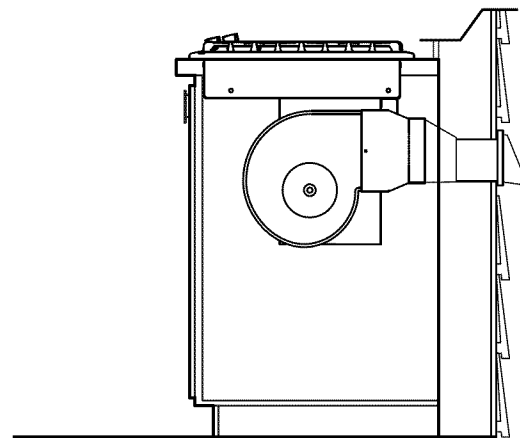
Figure 8 – CONDUIT À TRAVERS LE MUR
