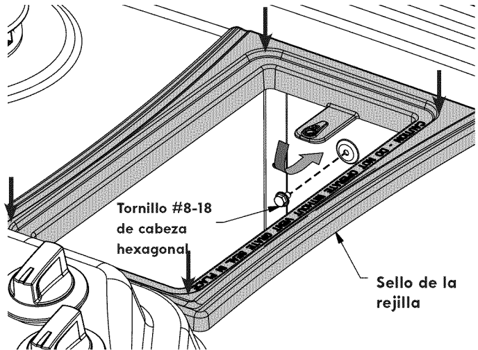
Figura 30 FIJACIÓN DEL SELLO DE LA REJILLA DE VENTILACIÓN – MODELO DE 30 PULGADAS
