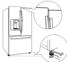
5 Nivellement et alignement de la porte.
