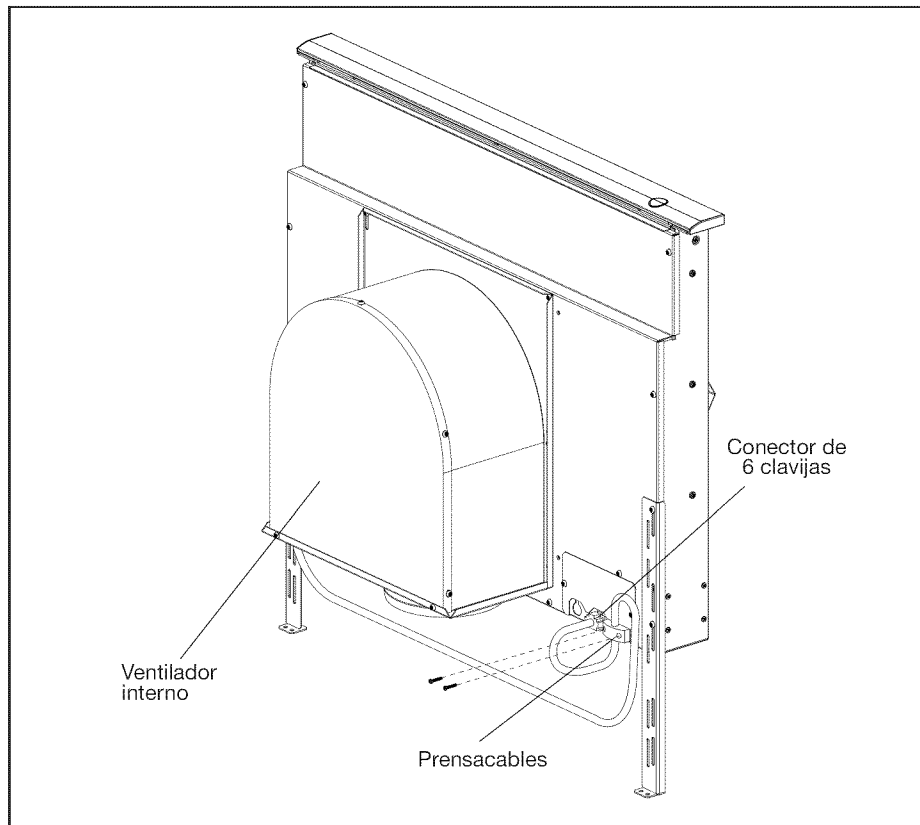
Fig. 9 – Ventilador interno
