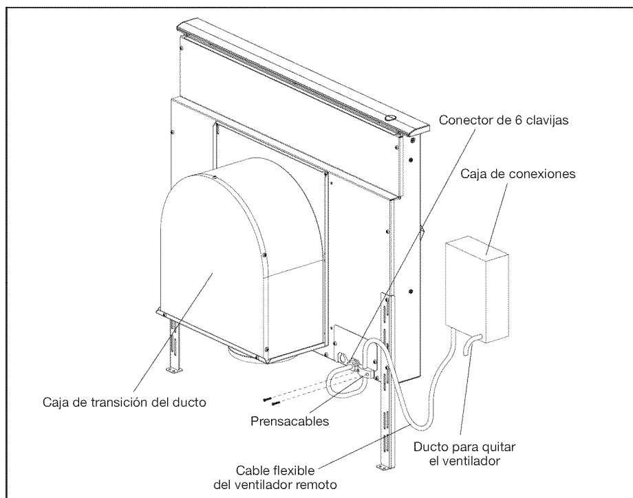
Fig. 10 – Ventilador remoto
