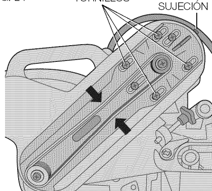
FIG. 24 TORNILLOS TORNILLO DE SUJECIÓN
