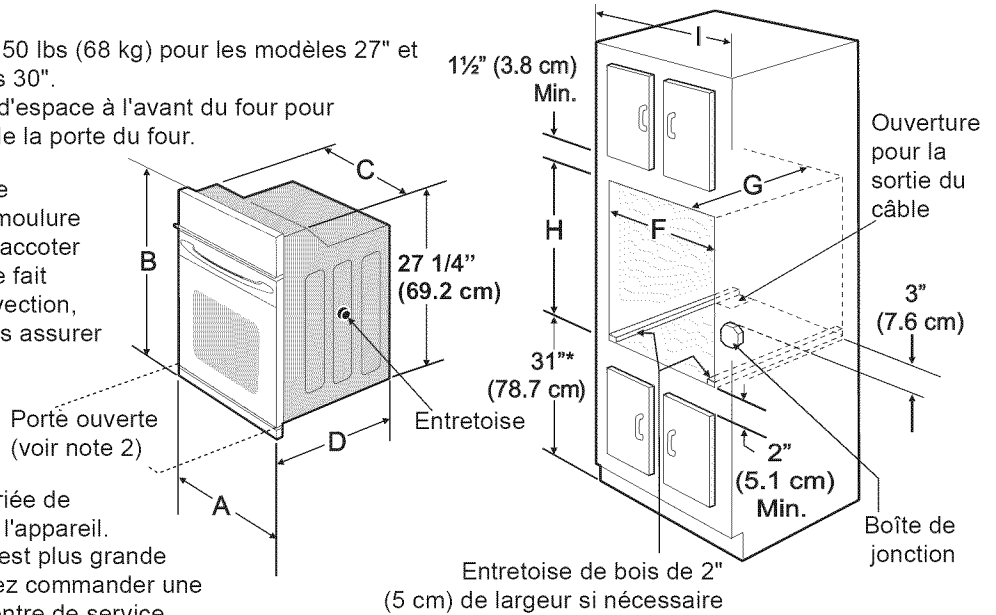
Figure 1 Fours encastrés simples 27" et 30" (Pour les fours encastrés doubles voir la figure 2)
