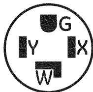
PRISE TYPIQUE 30 AMP POUR SÈCHEUSE
