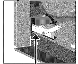
Verrou en position déverrouillée
