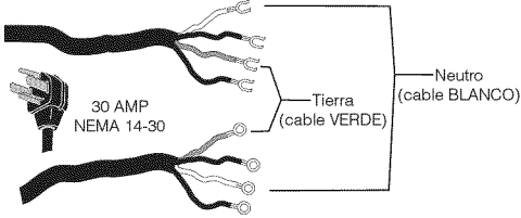
Receptáculo tetrafilar (tipo NEMA 14-30R)
