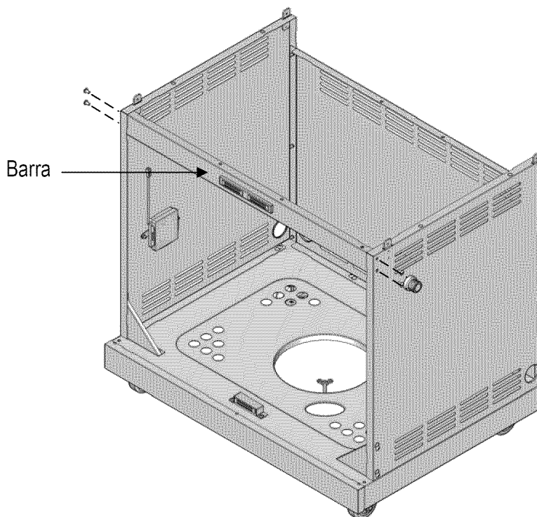
Tornillo de 3/16-24 x 3/8" Cant. 4
