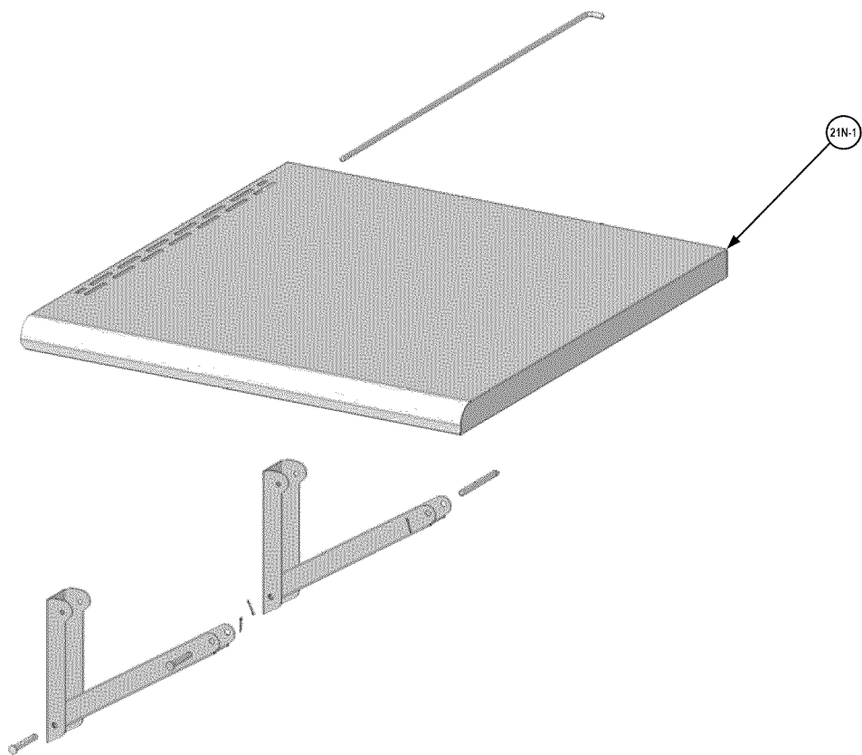
Mesa de ala: Diagrama con piezas expuestas
