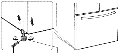
tournevis à tête plate (-) Molette
