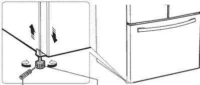
Destornillador de punta chata (-) Palanca de control chata (-)
