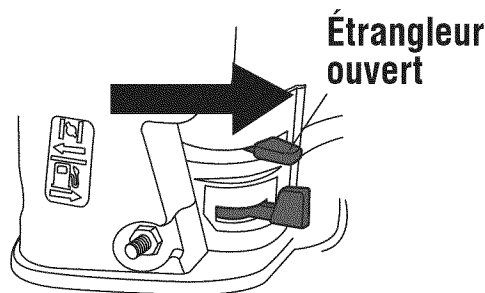
Figure 28 - Levier d'étrangleur
