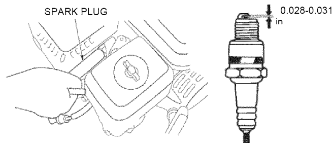
Figura 36 – Cambio de la bujía
