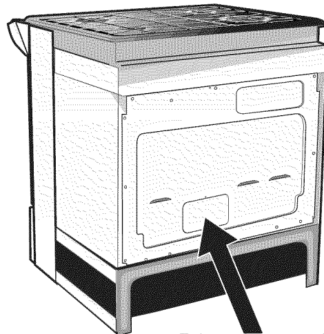
Enlevez le couvercle arrière pour accéder aux bornes du bloc de connexion de la cuisinière
