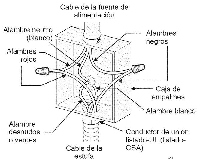
Figura 6 - 4 - Cable (Neutral) sistema eléctrico (Ejemplo: Caja de paso)
