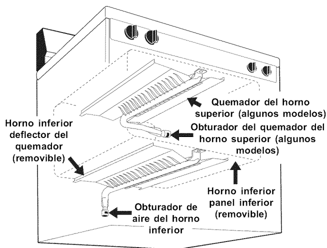
Fig. 20 - ubicaciones de los quemadores del horno
