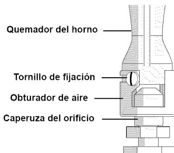
Fig. 21 - Obturador de aire típico del quemador del horno
