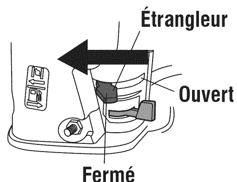
Figure 21 - Levier d'étrangleur
