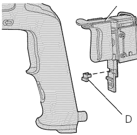
FIG. 3 SWITCH ASSEMBLY INTERRUPTEUR MONTAJE DEL INTERRUPTOR
