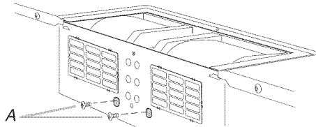
A. Vis (dans les trous décalés)
