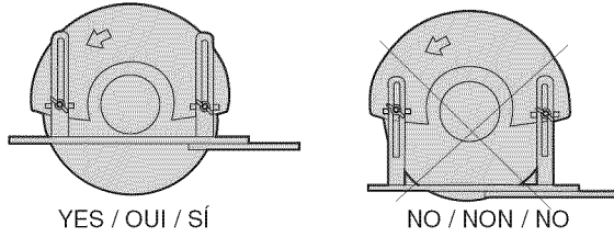
FIG. 6 METALS OR THIN MATERIAL MÉTAUX OU MATÉRIAUX MINCES METALES O MATERIAL FINO
