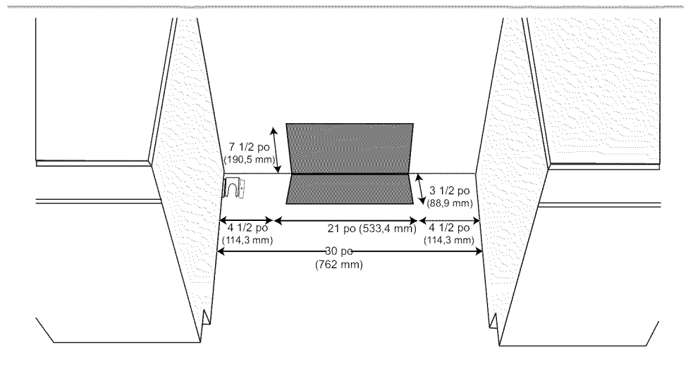
Figure 1: Dégagements de la surface de cuisson
