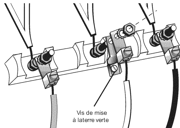
Figure 22: Conduit flexible à 3 fil compléte
