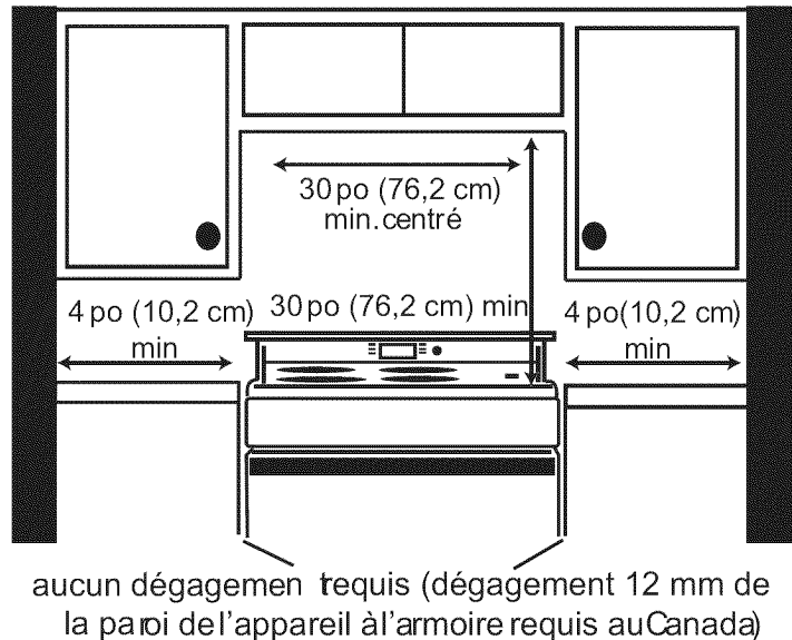
Figure 4: Préparation d'armoire
