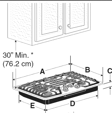
Dimensions de la plaque de cuisson
