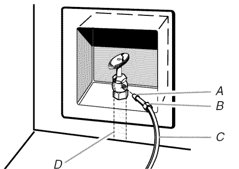
A. Bulbo B. Tuerca C. Tubería de cobre (al refrigerador) D. Línea de suministro doméstica ( \frac{1}{2} " como mínimo)
