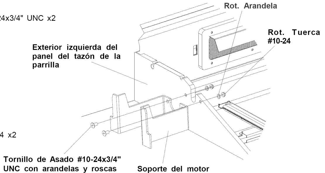
Rot. Arandela x2
