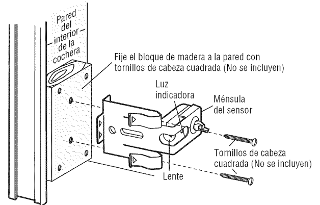
Figura 3 INSTALACIÓN EN LA PARED (LADO DERECHO)
