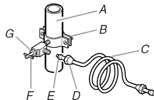
A. Canalisation d'eau froide B. Bride de tuyau C. Tube en cuivre D. Écrou de compression E. Manchon à compression F. Robinet d'arrêt G. Écrou de serrage
