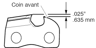
Figure 26 - Arrondir le coin avant du limiteur de profondeur
