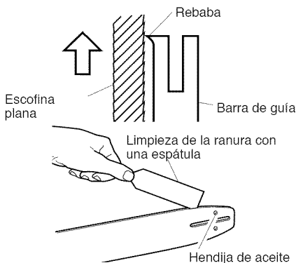
Figura 21 - Mantenimiento de la barra de guía
