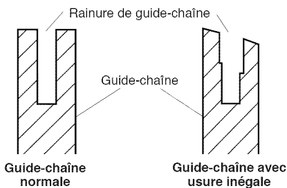
Figure 19 - Coupe transversale d'une guide-chaîne montrant une usure inégale
