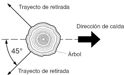
Figura 7 - Trayecto de retirada de un árbol
