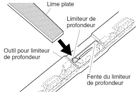
Figure 25 - Position de l'outil pour limiteur de profondeur sur la chaîne
