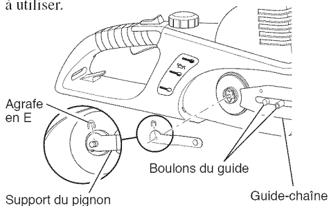
Figure 20 - Retrait de l'agrafe en E et du support de pignon
