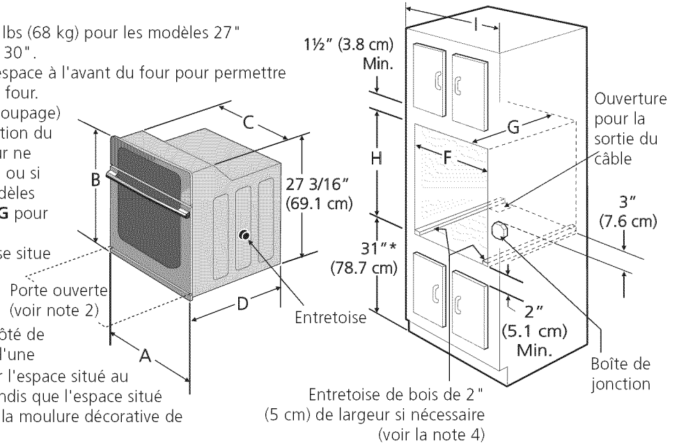
Figure 1 Fours encastrés simples 27" et 30" (Pour les fours encastrés doubles voir la figure 2)
