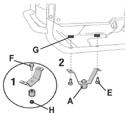
Fig 2-2: Pies del bastidor y parachoques de caucho
