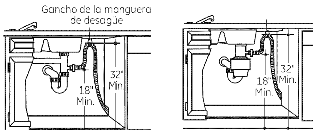
Instalación del eliminador de desechos
