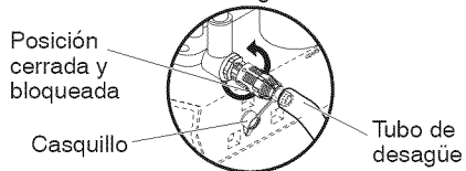
Válvula de desagüe del aceite
