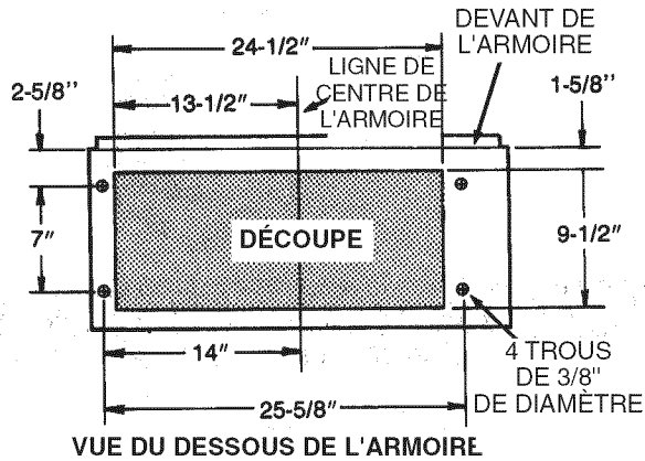
VUE DU DESSOUS DE L'ARMOIRE
