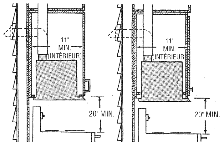
9 ARMOIRE À BASE LISSE
