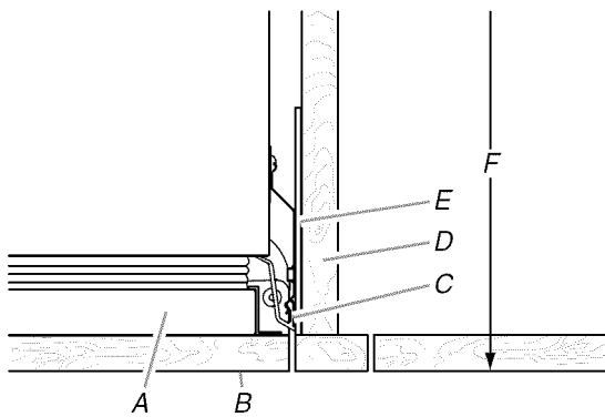
A. Puerta del refrigerador B. Panel de la puerta C. Moldura lateral D. Armario adyacente E. Soporte de la rejilla F. 25" (63,5 cm)
