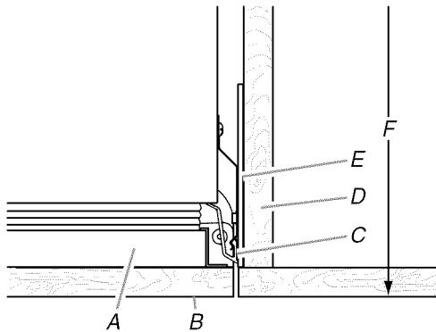
A. Puerta del refrigerador B. Panel de la puerta C. Moldura lateral D. Armario adyacente E. Soporte de la rejilla F. 25" (63,5 cm)
