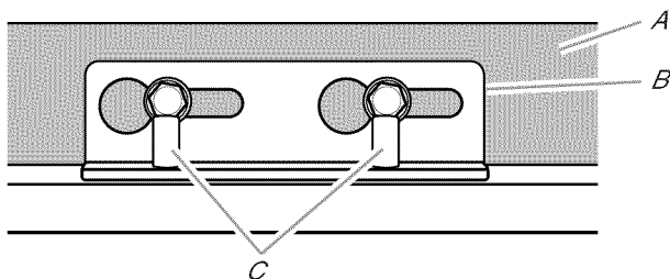
A. Panel de la puerta B. Soporte de montaje C. Pasadores de ajuste
