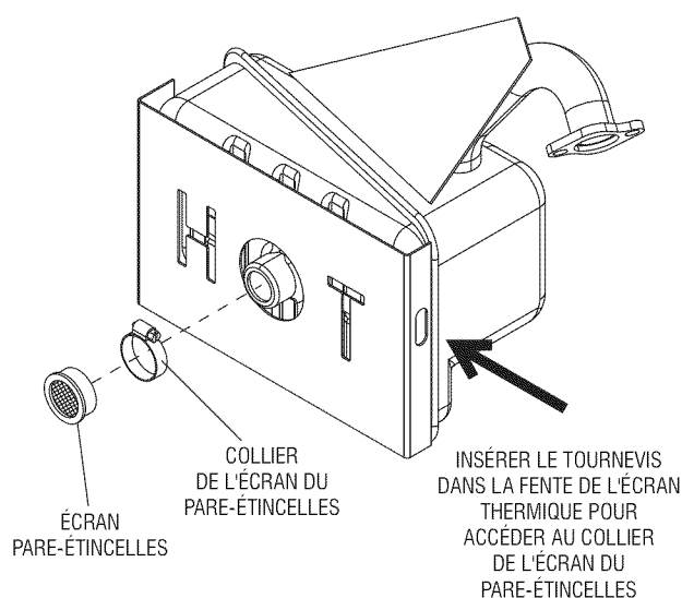
Schéma 14 - Pare-étincelles
