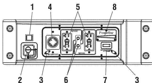
Schéma 3 - Commandes du générateur
