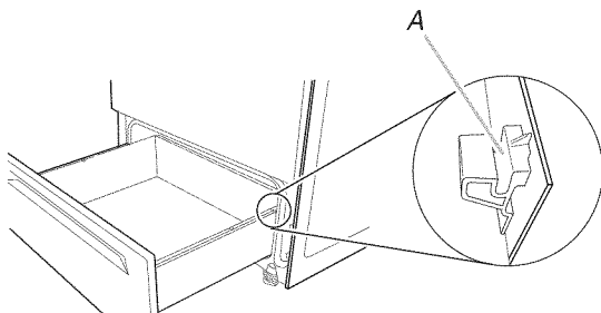
A. Engager la glissière du tiroir.
