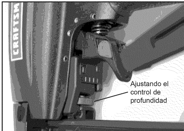
Figura 9- Ajustando el control de profundidad
