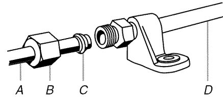
A. Canalisation jusqu'à la machine à glaçons C. Virole (achetée) B. Écrou (acheté) D. Canalisation d'alimentation en eau de la machine à glaçons (fournie)
