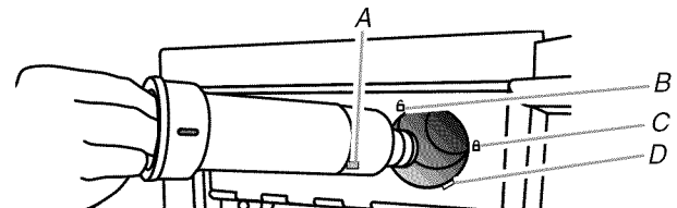
A. Tige d'alignement B. Symbole de déverrouillage C. Symbole de verrouillage D. Encoche dans le logement du module de commande
