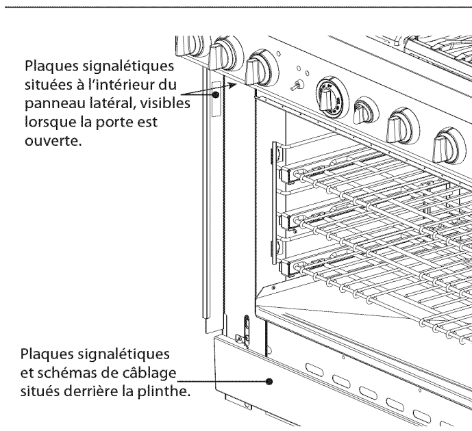
Figure 28 : Emplacement plaque signalétique et diagramme de câblage (porte du four non illustrée)
