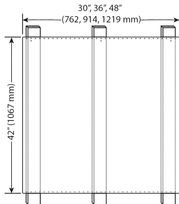
Figure 15 : Installation du dossieret de protection
