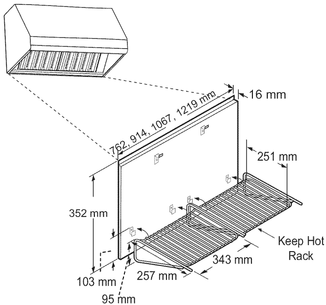
Figura 18: Estante guarda-caliente
