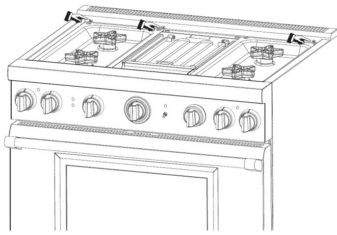
Figure 22 : Retrait des vis de la partie avant de la garniture d'îlot
