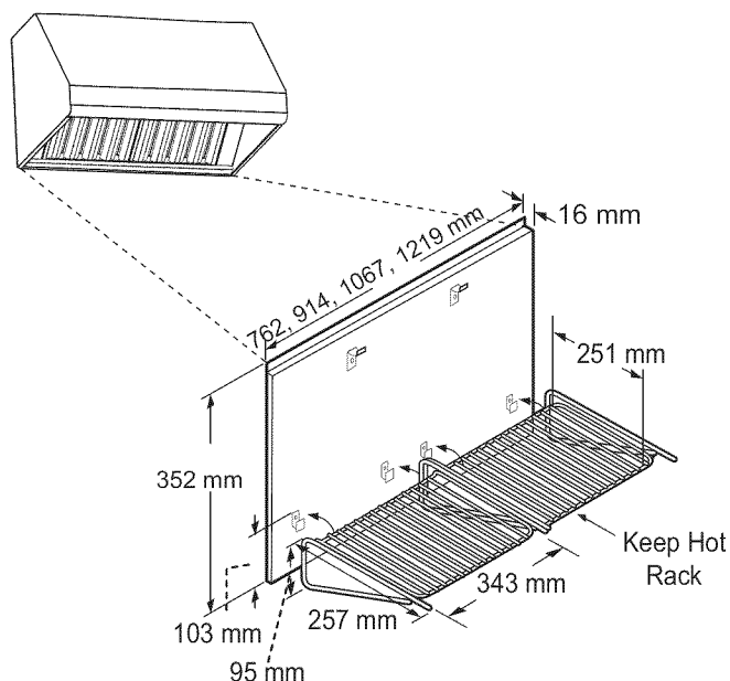
Figure 18 : Étagère garde-chaud
