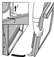
Figura 25: Para quitar la puerta de la hornilla:
