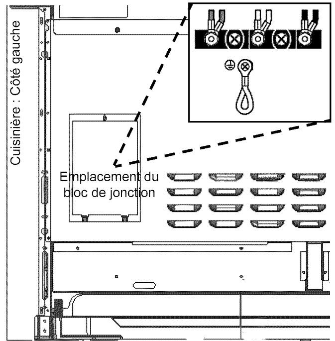
Figure 11 : Emplacement du bloc de jonction
