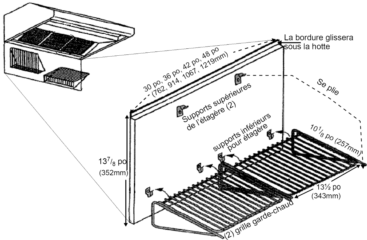
Figure 18 : Étagère garde-chaud
