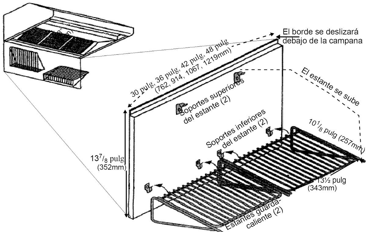
Figura 18: Estante guarda-caliente
