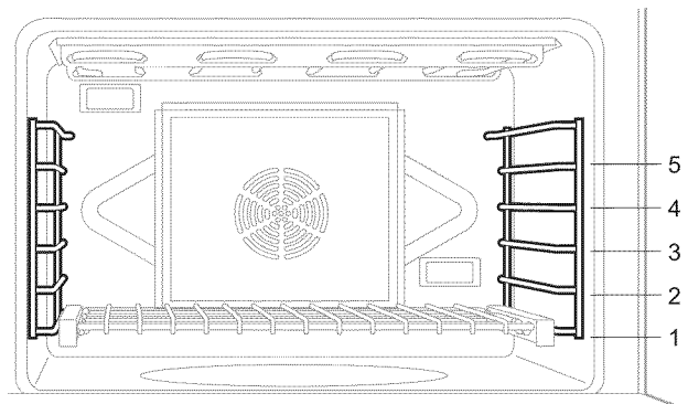
Figure 27 : Four principal au gaz avec positions des grilles
