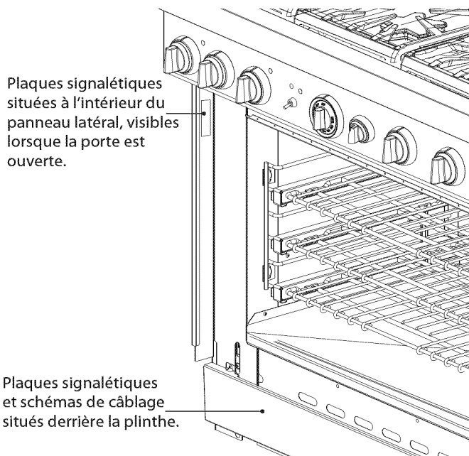
Figure 33 : Emplacement plaque signalétique et diagramme de câblage (porte du four non illustrée)
