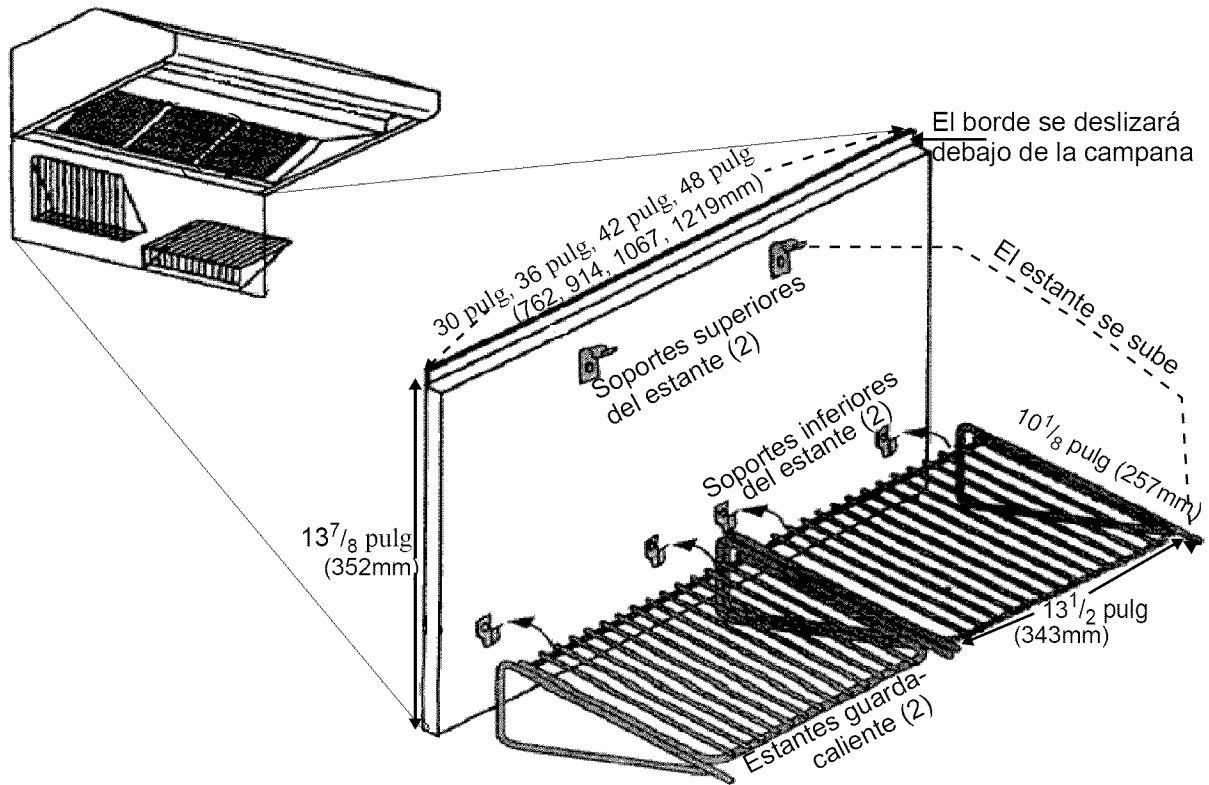
Figura 16: Estante guarda-caliente
