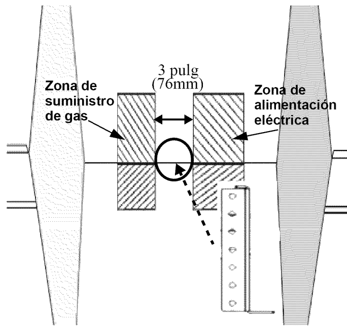
Figura 10: Ubicación para la instalación del dispositivo antivuelco
