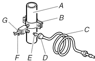
A. Canalisation d'eau froide B. Bride de connexion C. Tube de cuivre D. Écrou de compression E. Virole de compression F. Robinet d'arrêt G. Écrou de serrage
