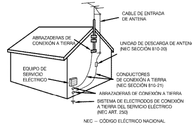
EJEMPLO DE CONEXIÓN A TIERRA DE LA ANTENA SEGÚN EL CÓDIGO ELÉCTRICO NACIONAL, ANSI/NFPA 70
