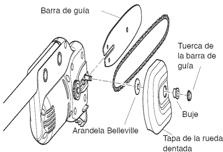
Figura 1 - Instalación de la barra guía
