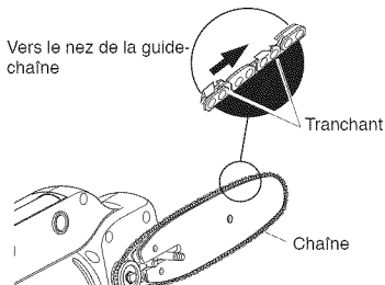
Figure 2 - Position de la chaîne
