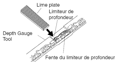
Figure 16 - Position de l'outil pour limiteur de profondeur sur la chaîne
