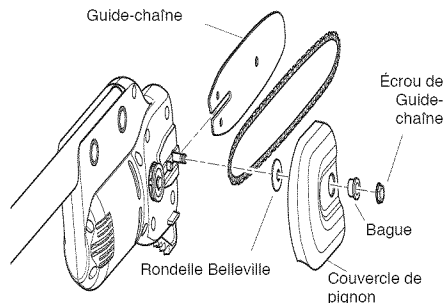
Figure 1 - Installation du guide-chaîne
