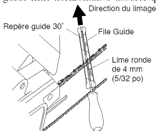
Figure 14 - Position de la lime et du guide lime sur la chaîne
