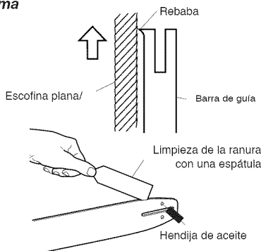
Figura 13 - Mantenimiento de la barra de guía
