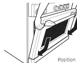
Bras de charnière Bord inférieur de la rainure Retrait
