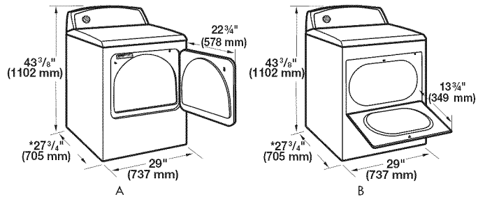
A. Porte à pivotement latéral à grande ouverture B. Porte rabattable à large ouverture
