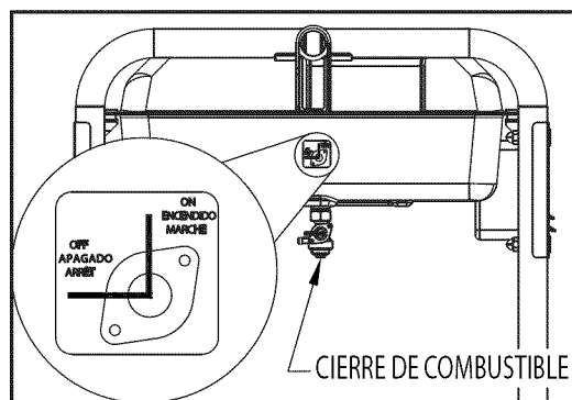
Figura 11 - Interruptor ON/OFF del motor
