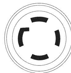
Schéma 7 - Prise 120/240 V c.a., 30 A
