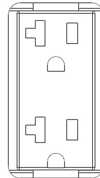
Figure 6 - 120 Volt AC, 20 Amp, Duplex Receptacle
