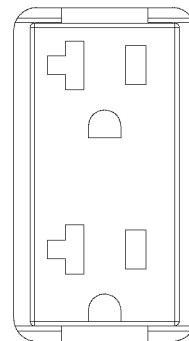
Schéma 6 - Prise double, 120 V c.a., 20 A
