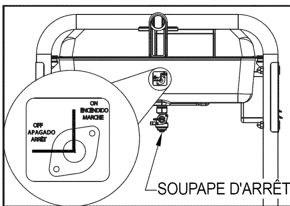
Figure 11 - Interrupteur ON/OFF du moteur
