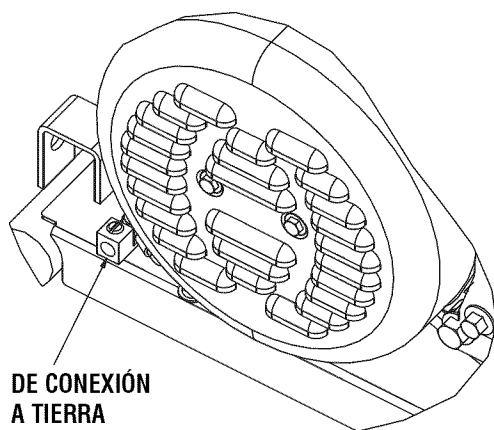
Figura 8 - Conexión a tierra del generador
