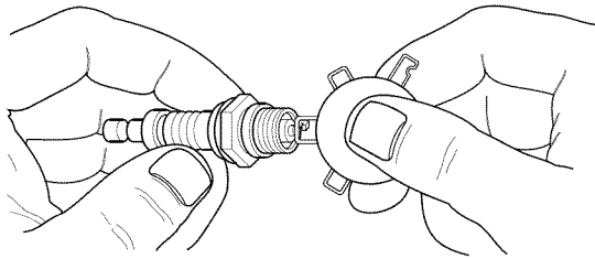
Figura 14 - Espaciamiento de la bujía
