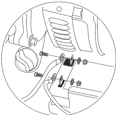
Figura 15 - Conexiones de la batería
