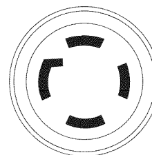
Figura 7 - Receptáculo de 120/240 VAC, 30 Amp
