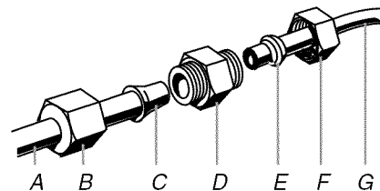
A. Conduit d'eau vers le réfrigérateur
