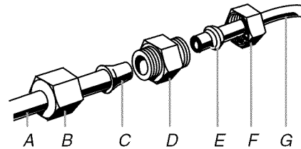
A. Tubería de agua del refrigerador B. Tuerca (provista) C. Bulbo
