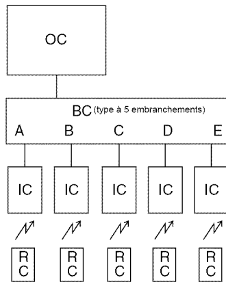
2-2. Type à 5 embranchements uniquement
