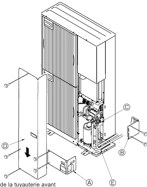
A Couverture de la tuyauterie avant B Couverture de la tuyauterie C Vanne d'arrêt D Panneau de service E Rayon de cintrage : 100 mm - 150 mm [3-15/16" - 5-7/8"]
