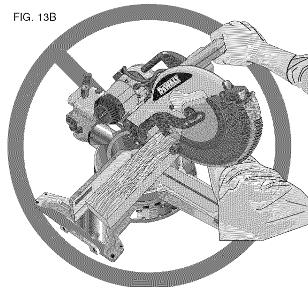
COUPE INADÉQUATE
