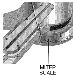
FIG. 6 MITER POINTER
