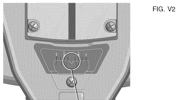
LE REPÈRE MICROMÉTRIQUE DE \frac{1}{4} ° S'ALIGNÉ AVEC LE REPÈRE DE DEGRÉ ENTIER LE PLUS PRÈS SUR L'ÉCHELLE À ONGLETS (ONGLET DROIT DE 24,5°)
