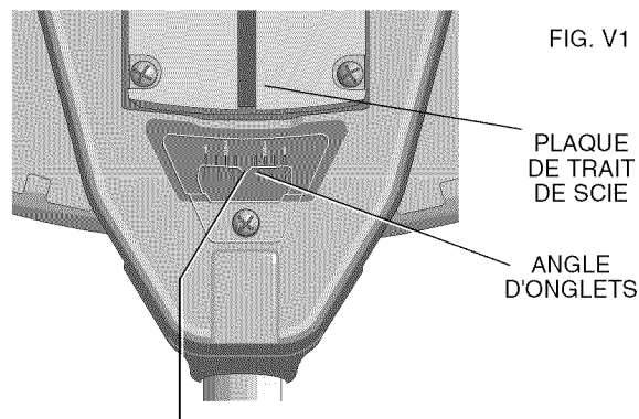
LE REPÈRE CENTRAL DE L'ÉCHELLE À VERNIER S'ALIGNÉ AVEC L'ANGLE ENTIER VOULU SUR L'ÉCHELLE À ONGLETS (ONGLET DROIT À 24°)
