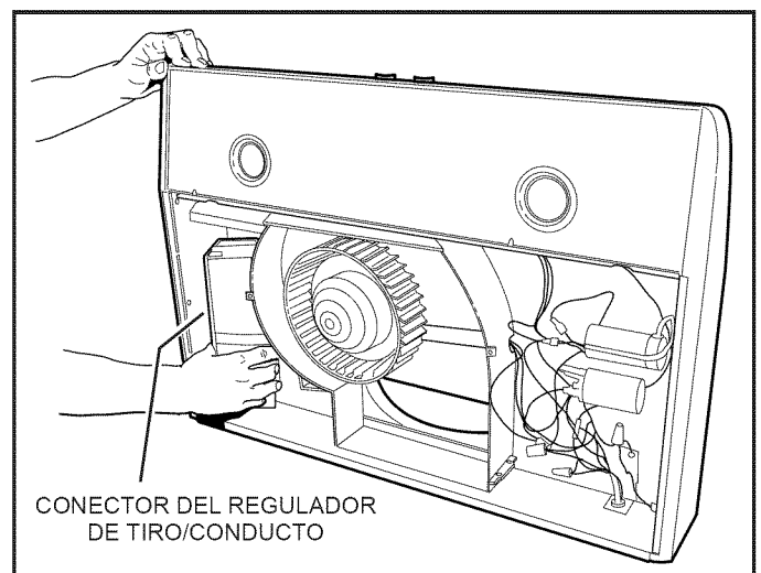
5 Quite el conector del regulador de tiro/conducto y bolsa de piezas del interior de la campana.
