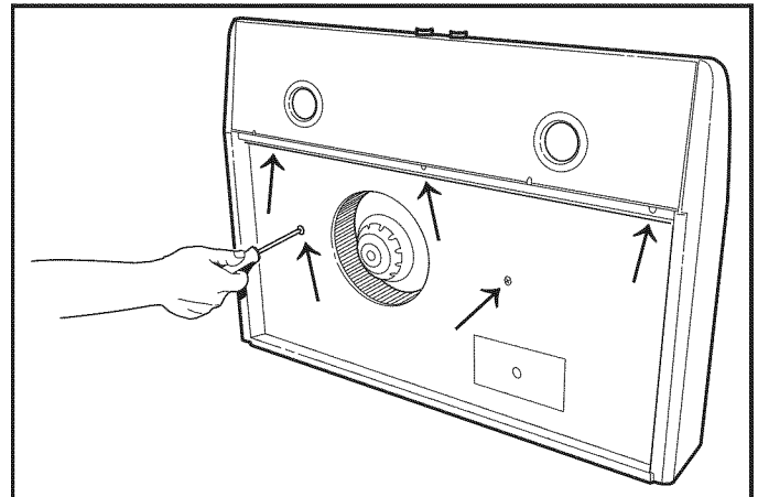
4 Enlevez le panneau inférieur maintenu par cinq (5) vis.
