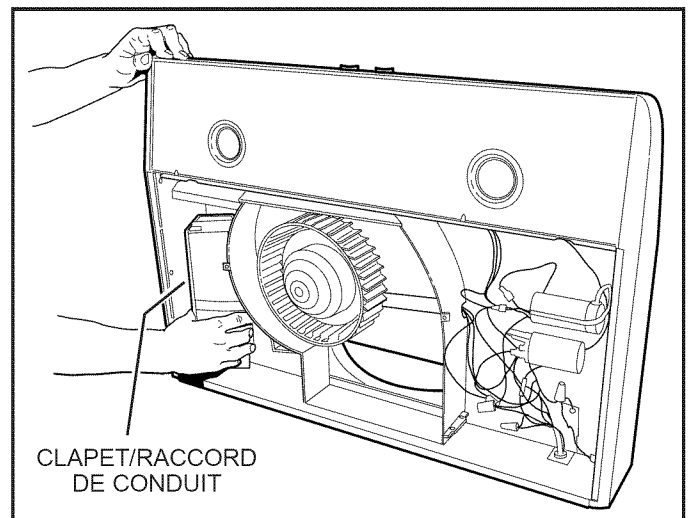
5 Enlevez le clapet/raccord de conduit et sac de pièces à l'intérieur de la hotte.
